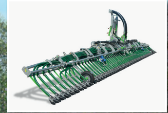
PENDISLIDE PRO Schleppschuhverteiler 120/48PS2
