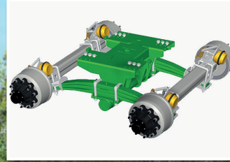
Roll-Over Boggie mit Nachlaufachse
