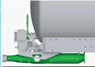
Schneckenpumpe mit Steinfangkasten und Vorausrüstung für Front-Jumbo
